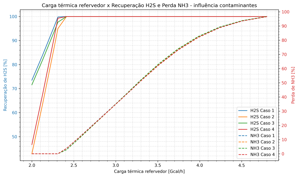
Figura 3: Carga térmica x recuperação de \text{H}_2\text{S} e perda de \text{NH}_3
